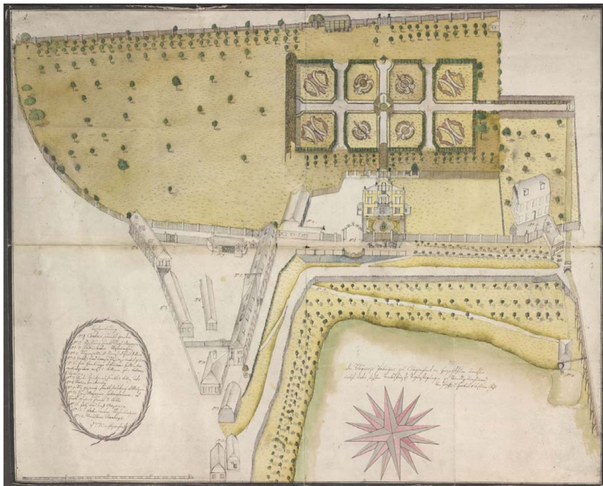
Plán továrny na výrobu běloby olovnaté v Klagenfurtu (NA, SMP, nezpracovaná část) 1775; rukopisná, barevná; německy; 62x51 cm; 1:40 (= 180 mm); průsvitka – C&I Honig
