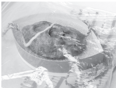
Obr. 9 Zabalení pečeti do plastové fólie pro omezení odpařování rozpouštědla
