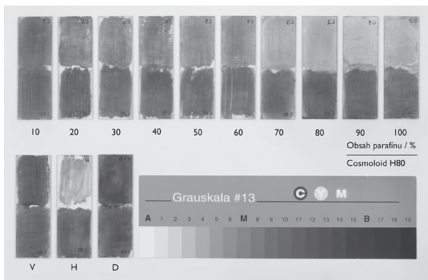
Obr. 5.1 Odolnost směsí Cosmoloid H80/parafín 62400 v různých poměrech vůči povrchovému znečištění. Srovnávací materiály: V = včelí vosk novodobý, H = včelí vosk hydrogenovaný (model historického vosku), D = včelí vosk s přísávkem 10% damarové pryskyřice [11]
