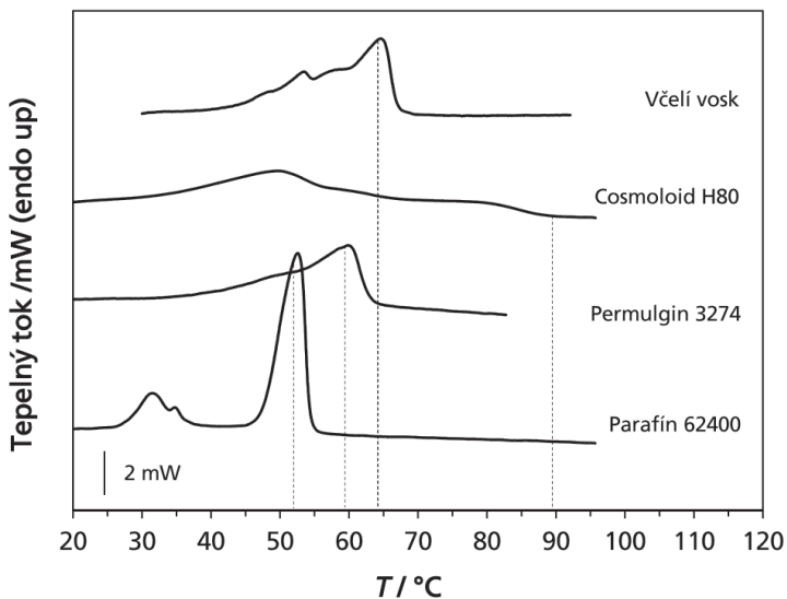
Obr. 3.1 Kalorimetrické ohřevové křivky vybraných vosků
