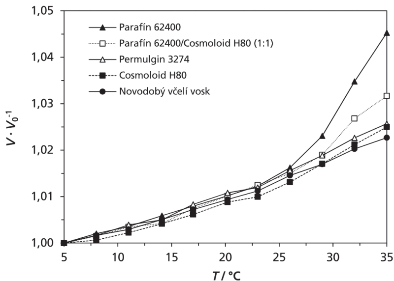
Obr. 2.1 Objemová teplotní roztažnost vybraných vosků a směsí. Významná je odchylka u parafinu při teplotách převyšujících cca 30^\circ\text{C}
