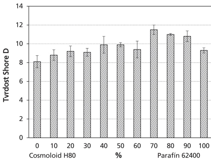
Obr. 1.2 Závislost tvrdosti Shore D na složení směsi vosku Cosmoloid H80 a parafinu 62400 [11]
