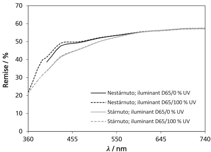
Obr. 8.6 Remisní křivky nestárnutého a stárnutého vosku cerezínového typu Permulgin 3274 (Koster Keunen). Stárnuté vzorky byly exponovány UV/VIS záření ve smyslu normy ISO 5630-7. Patrné je vyhasnutí UV fluorescence a žloutnutí po stárnutí
