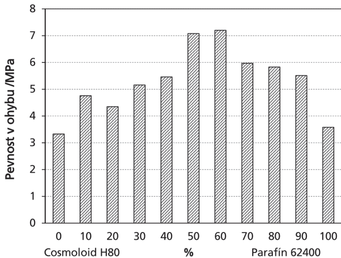
Obr. 1.1 Závislost pevnosti v ohybu na složení směsi vosku Cosmoloid H80 a parafinu 62400 [11]
