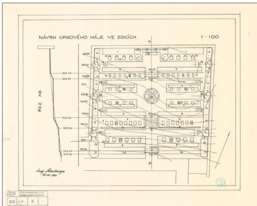
Řez resppektive půdorysný řez – návrh urnového háje ve Zdicích, (Archiv NZM OF Josef Miniberger, inv. č. 838/V/108)
