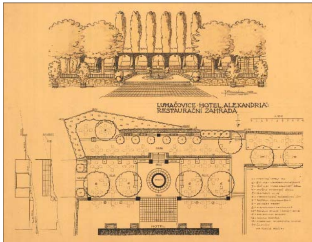
Půdorys – Luhačovice, hotel Alexandria, restaurační zahrada (Archiv NZM OF Josef Kumpán, inv. č. 527/V/Z/369)
