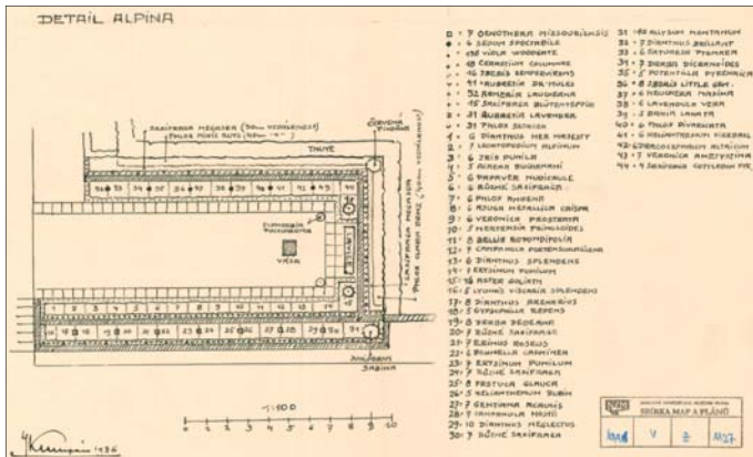
Detail – osazovací plán – detail alpina, (Archiv NZM OF Josef Kumpán, inv. č. 1991/V/Z/1127)
